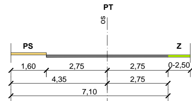
Profil A-A
