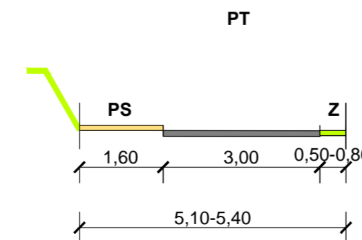
Profil B-B
